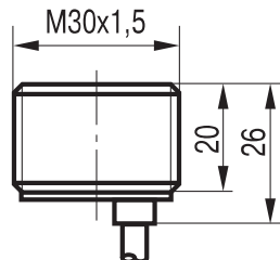
Габаритный чертеж
